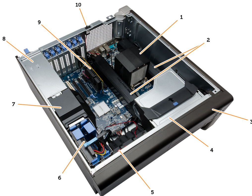
איור 1. מבט מבפנים על מחשב ה-T3610
